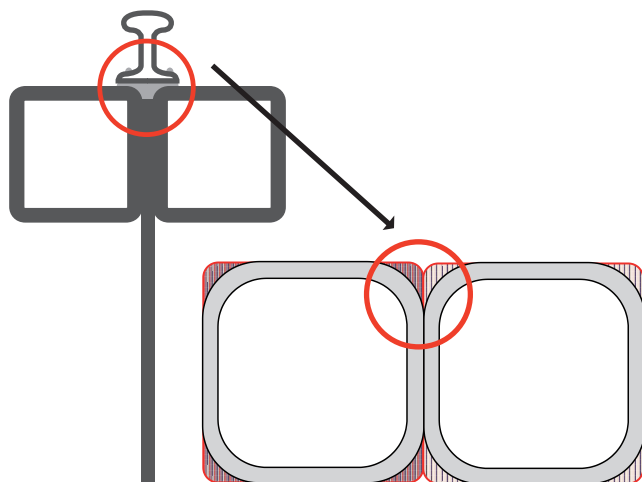
Vorteile Anwendung - Kranbahn
